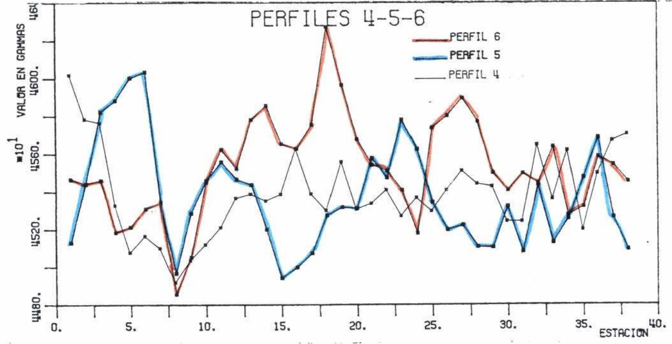
Figura nº 11. Perfiles magnetometria
