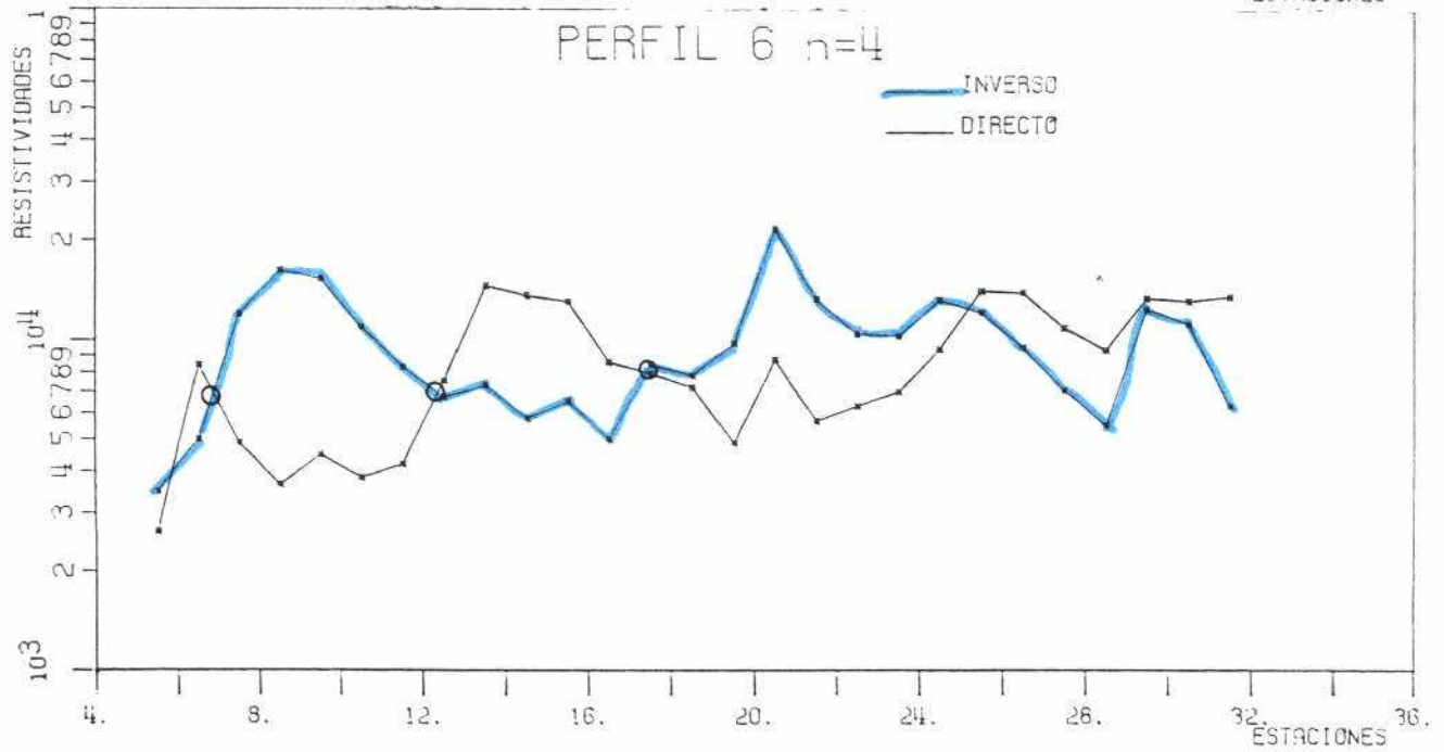
Figura. 8. Calicata trielectrónica combinada. Perfil 6
