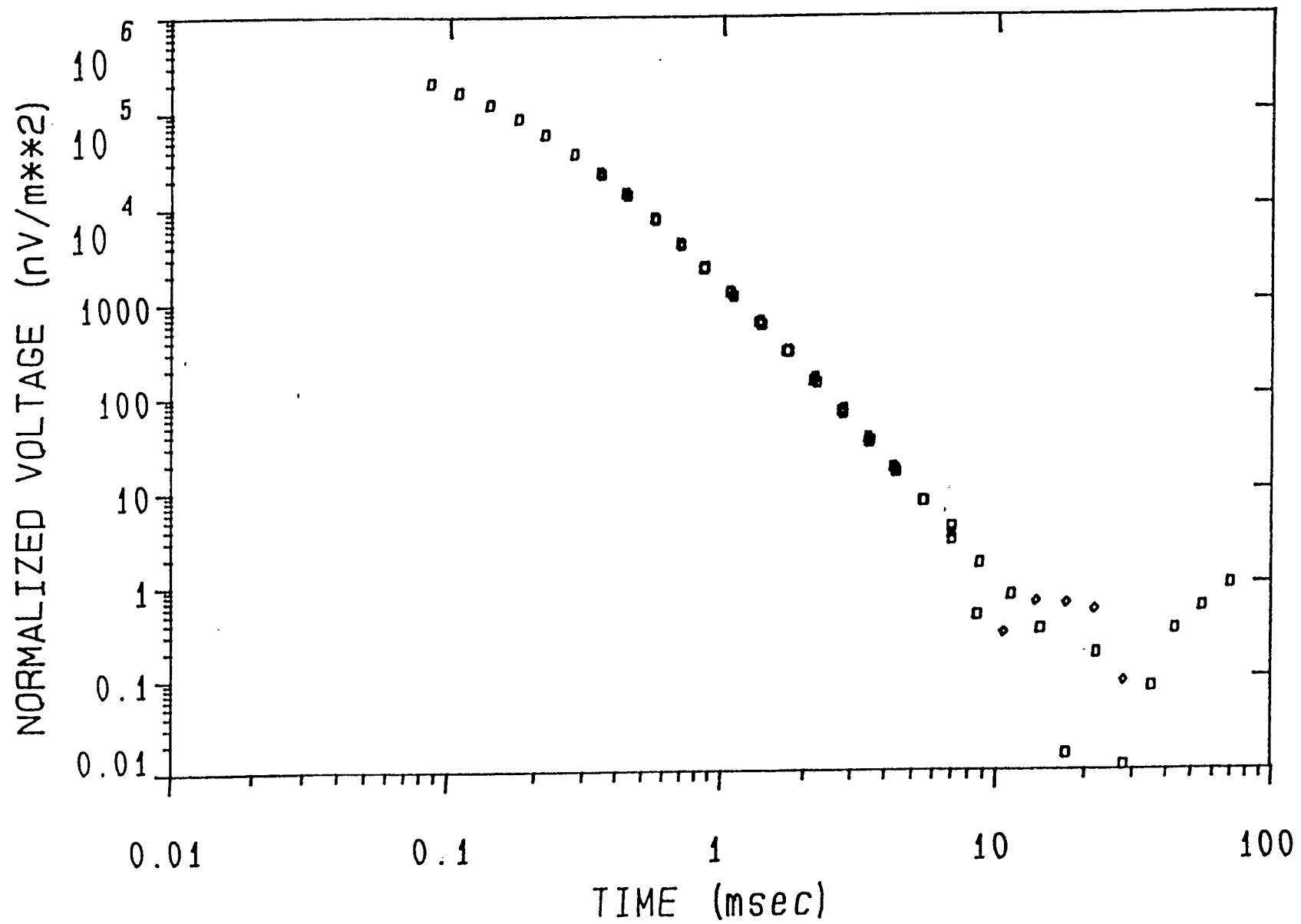
Fig. 12.- Ejemplo de respuesta de un medio resistivo en la curva de potencial normalizado.
