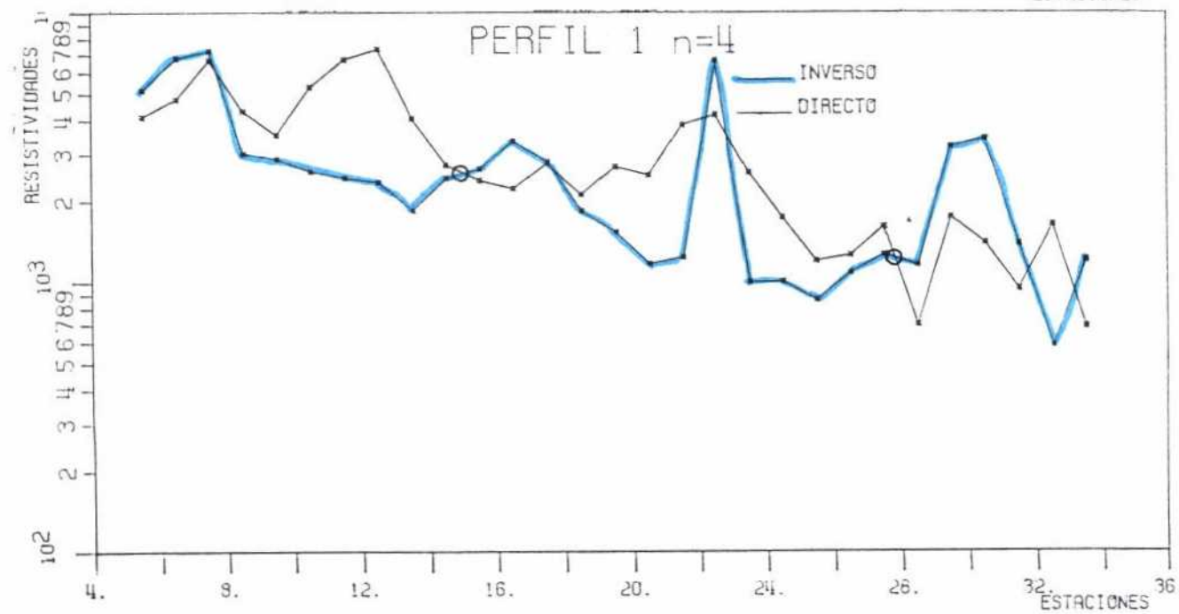
Figura nº 3. Calicata trieléctrica combinada. Perfil 1
