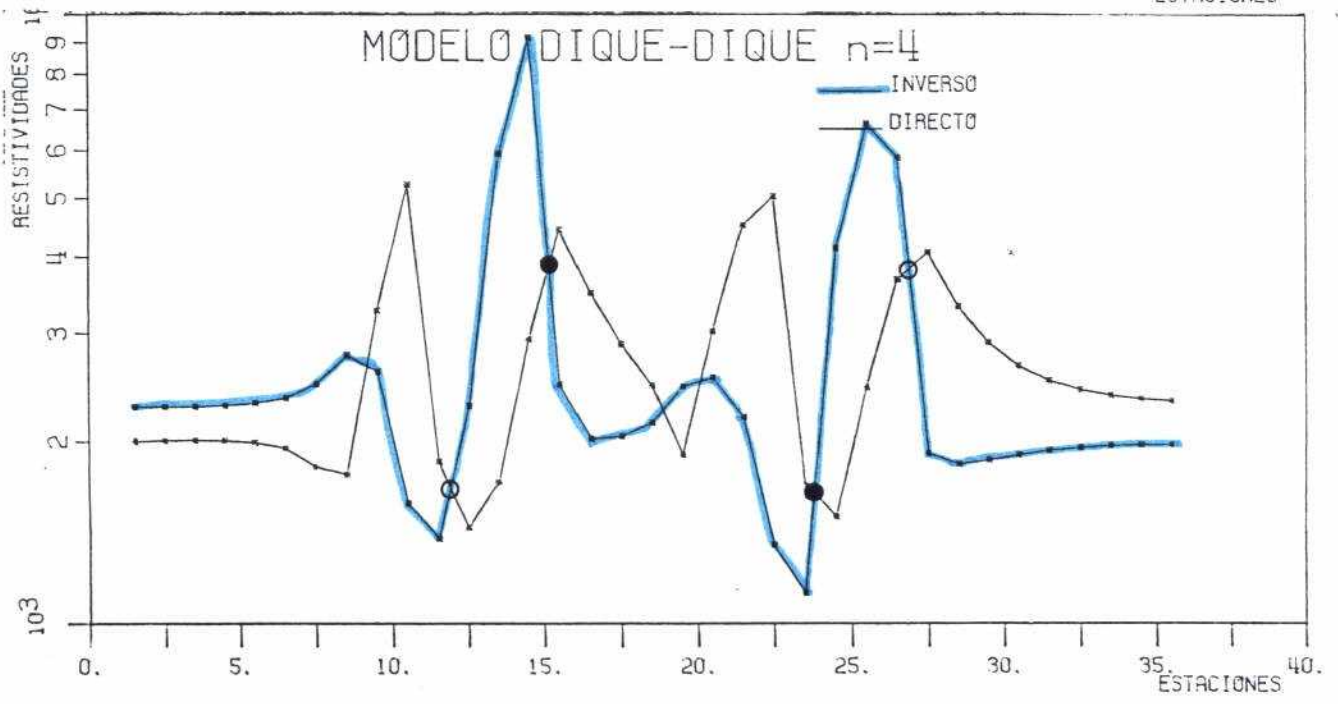
Figura nº 2. Calicata trieléctrica combinada sobre el modelo dique-dique para n=1, 2 y 4
