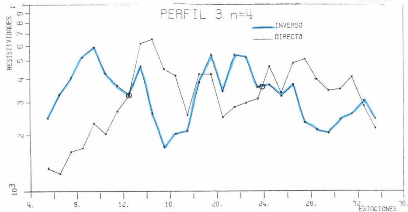
Figura nº 5. Calicata trielectrónica combinada. Perfil 3
