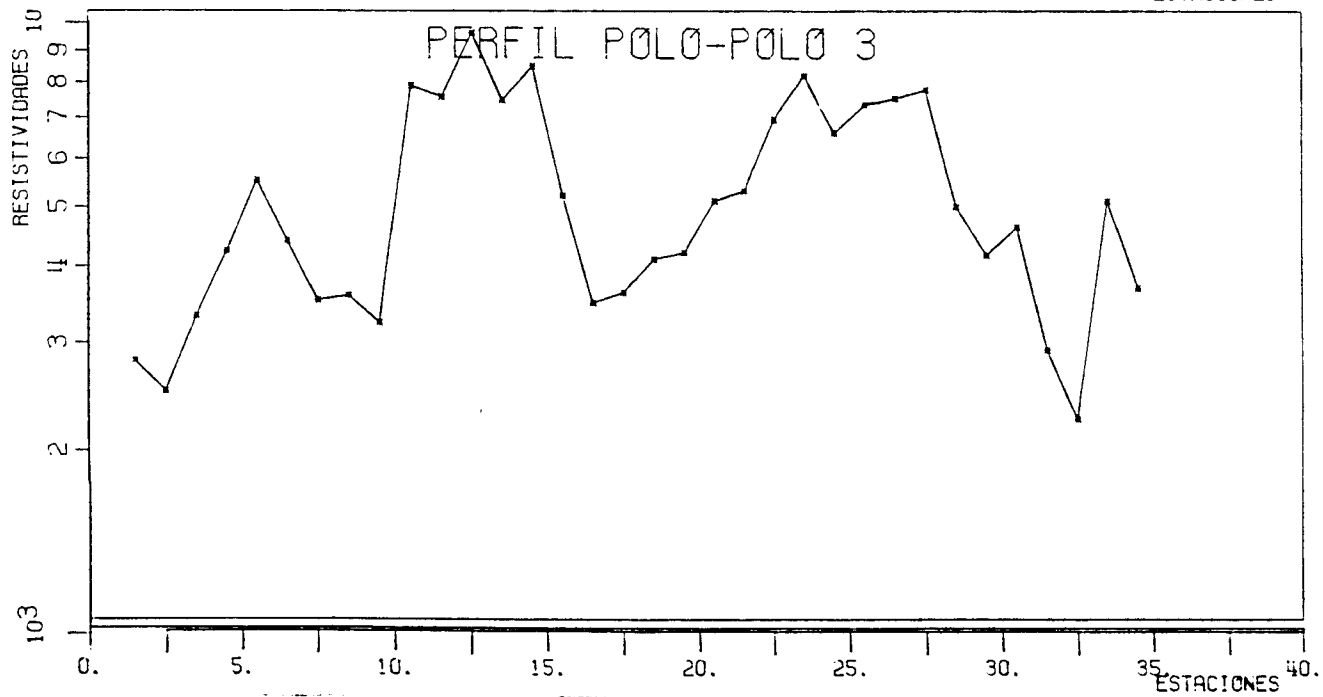
Figura nº 9. Perfiles polo-polo 1, 2 y 3
