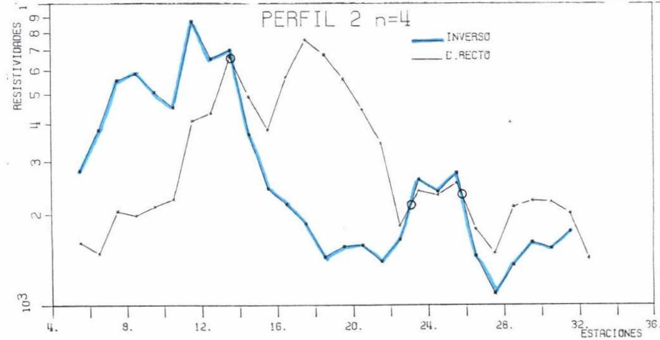
Figura n° 4. Calicata trielectrónica combinada. Perfil 2
