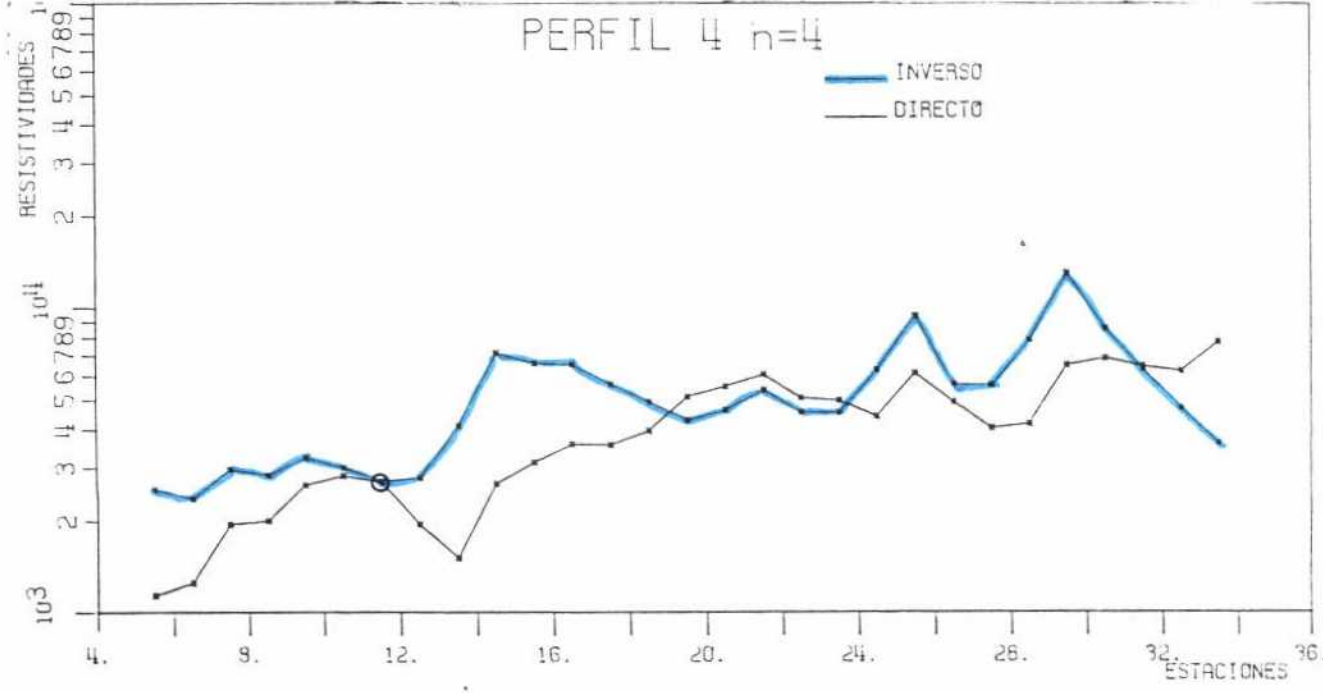
Figura nº 6. Calicata trieléctrico combinada. Perfil 4
