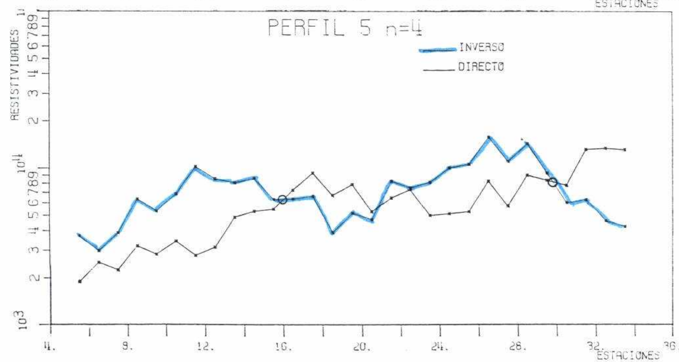
Figura 7. Calicata trieléctrica combinada. Perfil 5
